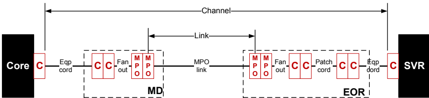
Exemple de calcul FO DC
