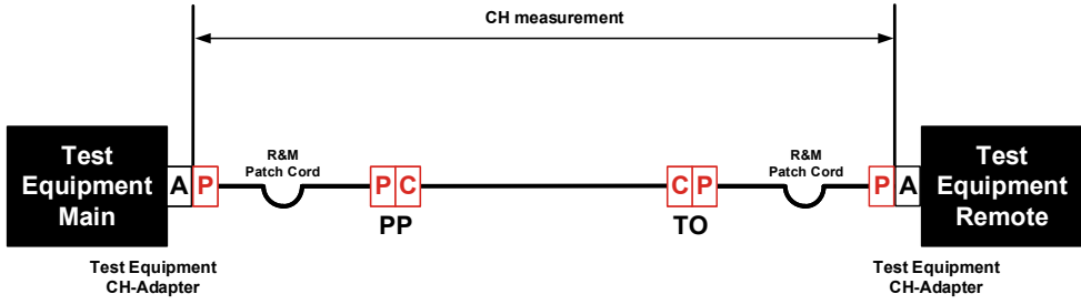
Exemple de lien de test CH
