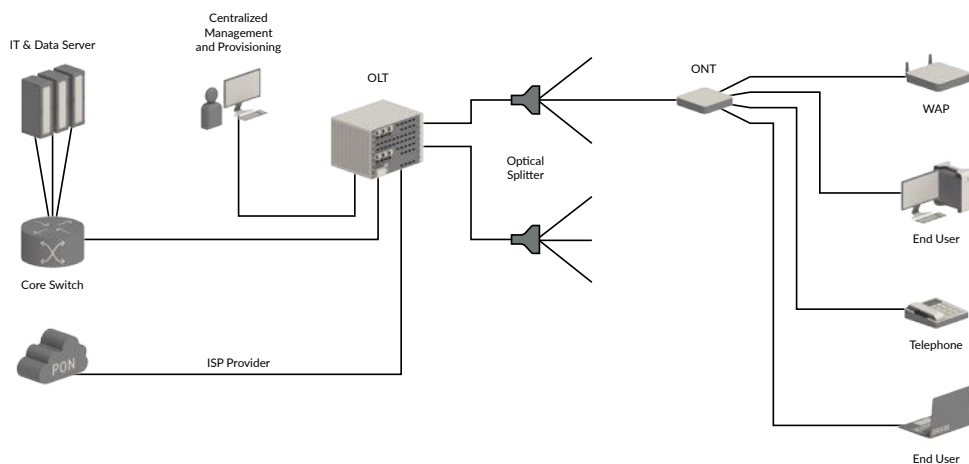
Schéma principal POLAN
