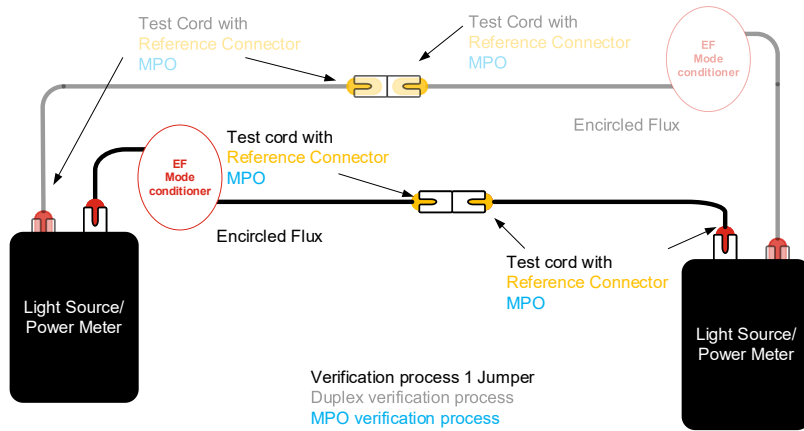
Vérification de la méthode «un cavalier»
