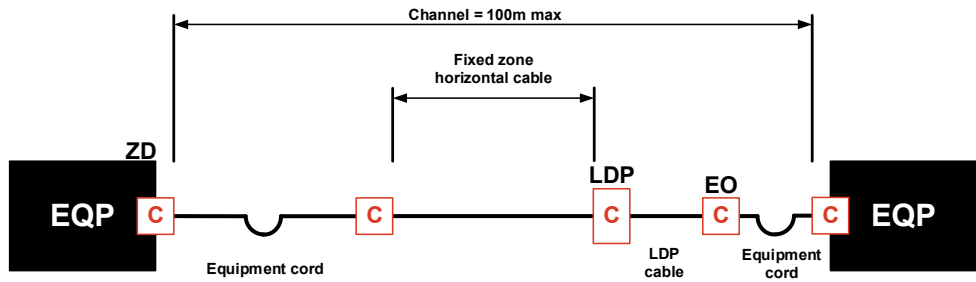
Interconnect-LDP-Modèle EO
