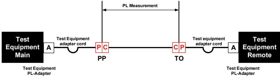
Exemple de lien de test PL
