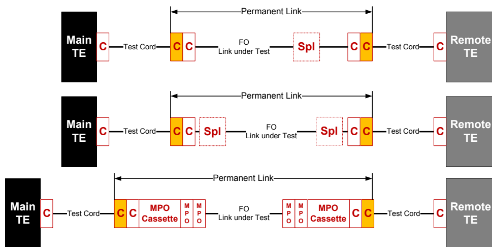
Câblage FO Configuration de la liaison permanente
