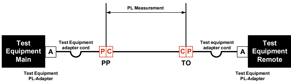
Exemple de test PL
