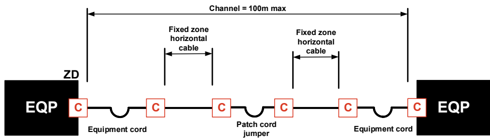
Modèle BtB interconnect
