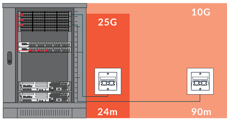
Restrictions de longueur Compatible 25G
