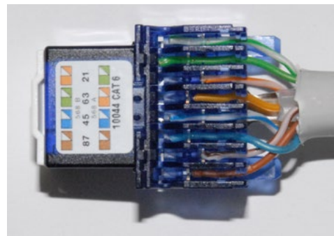
Câblage incorrect
