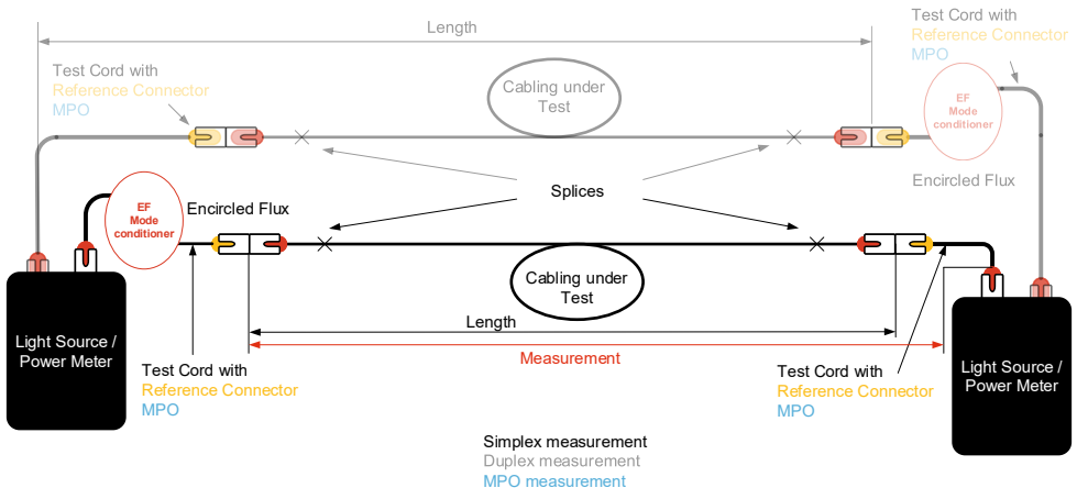
Mesure d'un PL
