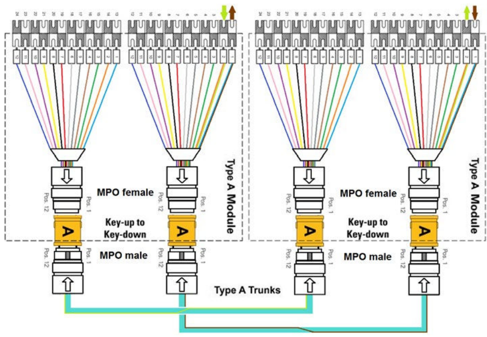
Méthode de polarité MPO A fan-out
