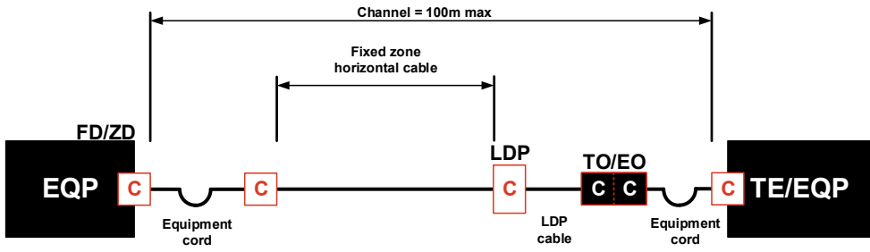
Interconnect LDP EO modèle avec un coupleur RJ45
