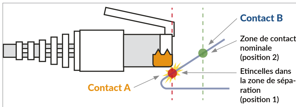
Étincelle lors de la déconnexion sous charge
