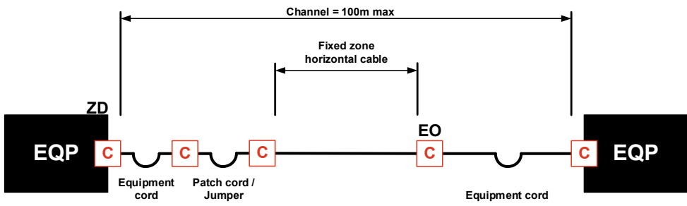
Cross connect-Modèle EO
