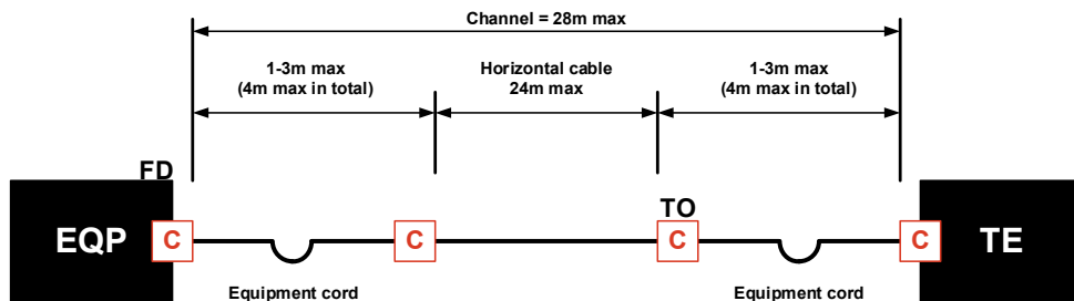
Représentation schématique de Cat. 8.1 avec spécification de la longueur
