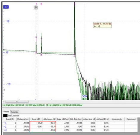
Mesure conventionnelle B vers A
