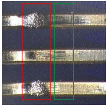
Bonne conception des contacts
