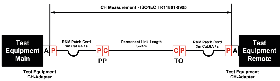
Exemple de test 25G
