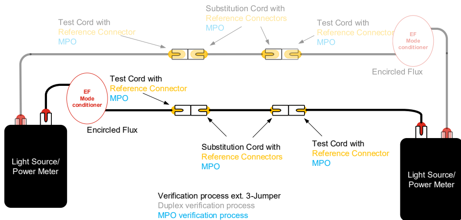
Vérification de la méthode «3-cavaliers étendus»
