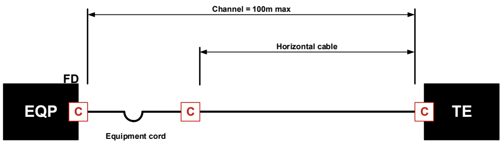
Modèle un conencteur OC
