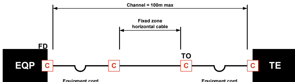
Interconnect Modèle-TO
