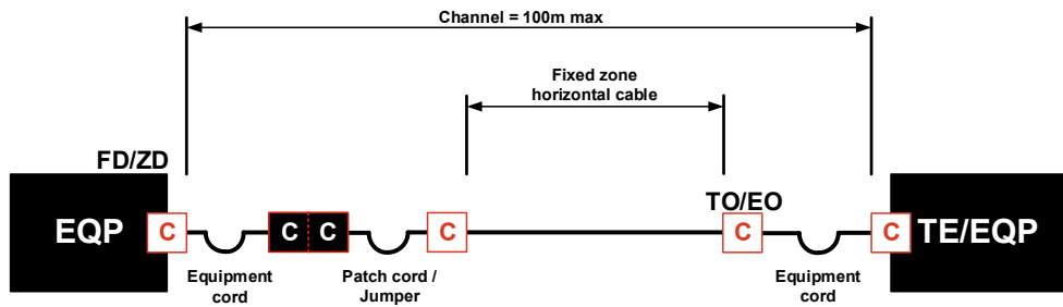
Connexion croisée modèle TO/EO avec coupleur RJ45
