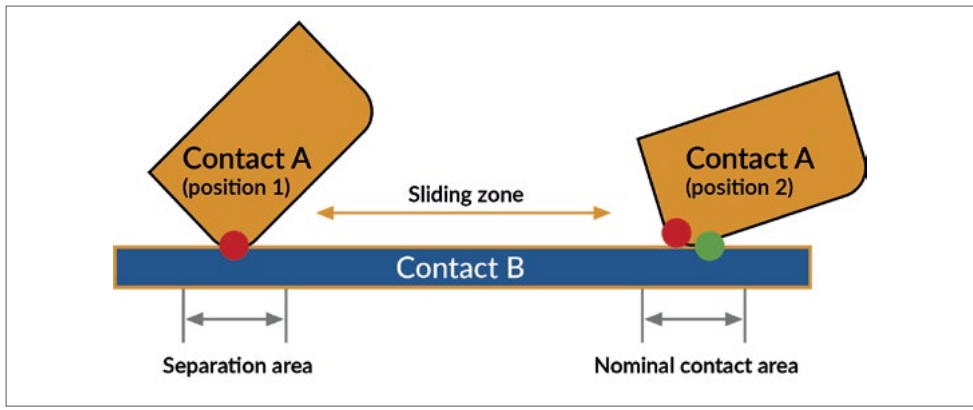
Point de contact de déplacement pendant le processus d'enfichage
