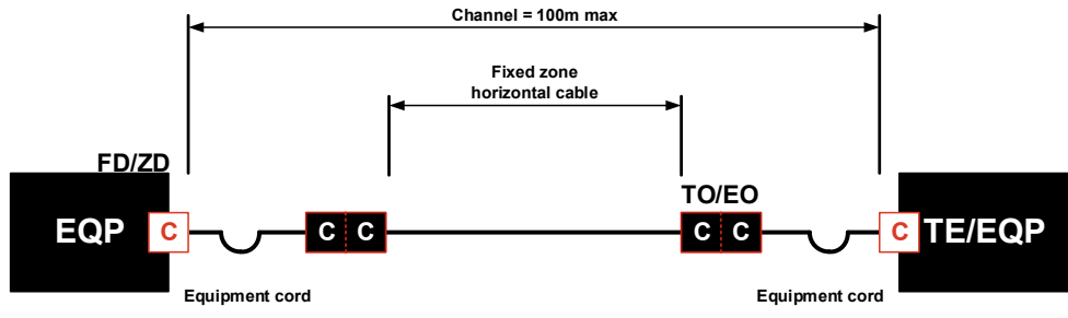
Interconnect TO/EO modèle avec coupleur RJ45
