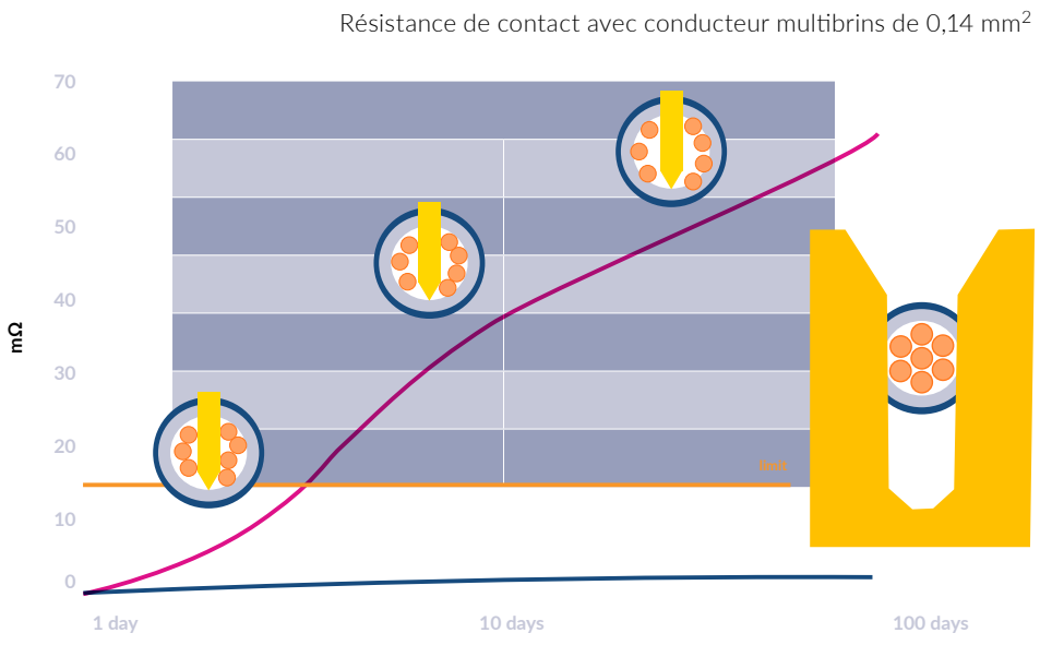
Comportement de résistance
