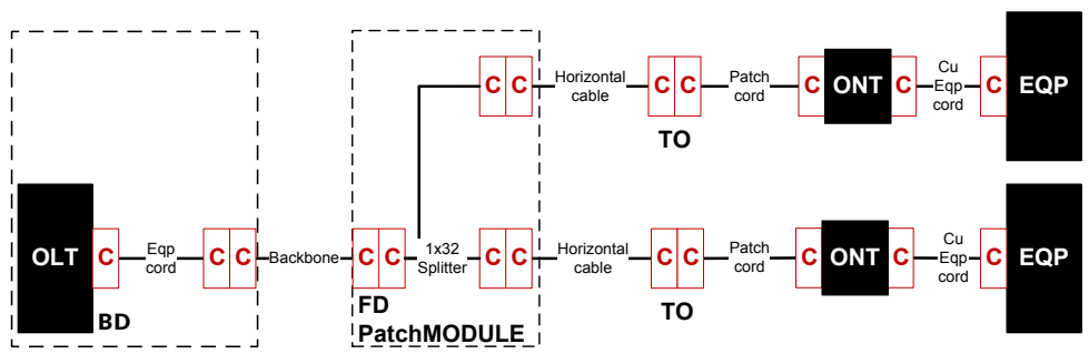
Exemple de calcul POLAN
