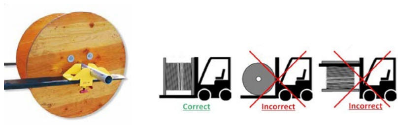
Bobine de déchargement avec barre Procédure de levage correcte
