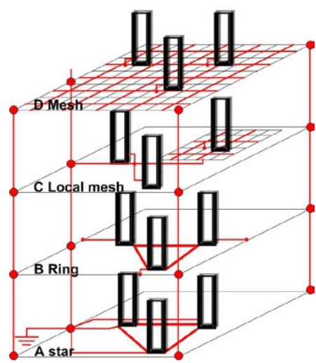
EN50310 Recommandé
