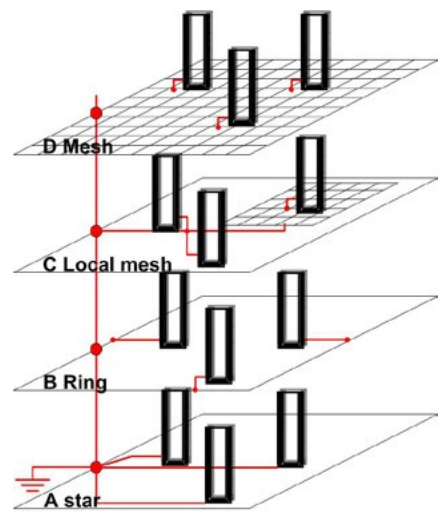
EN 50310 Minimum
