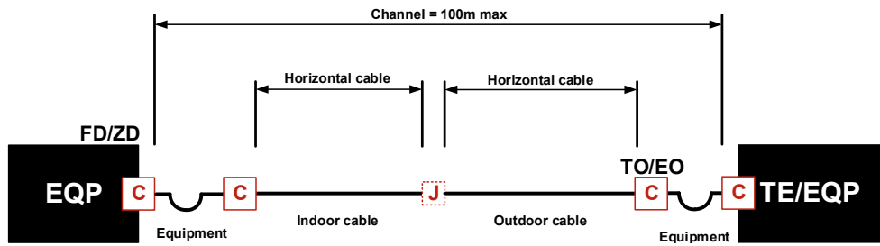
PL couplé MPTL intérieur/extérieur avec coupleur de câble
