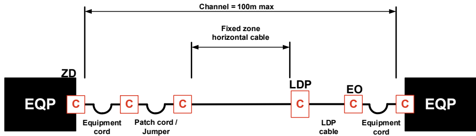
Cross connect-LDP-Modèle EO
