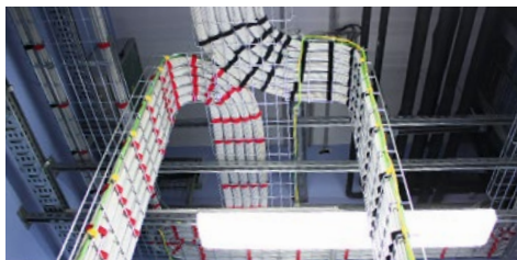
Installation correcte des colonnes montantes verticales
