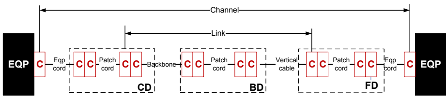
Exemple de calcul FO OC
