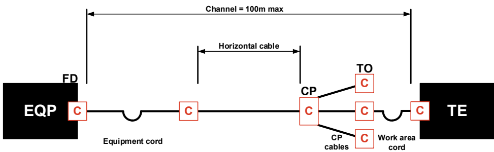
Interconnect-Modèle CP-TO
