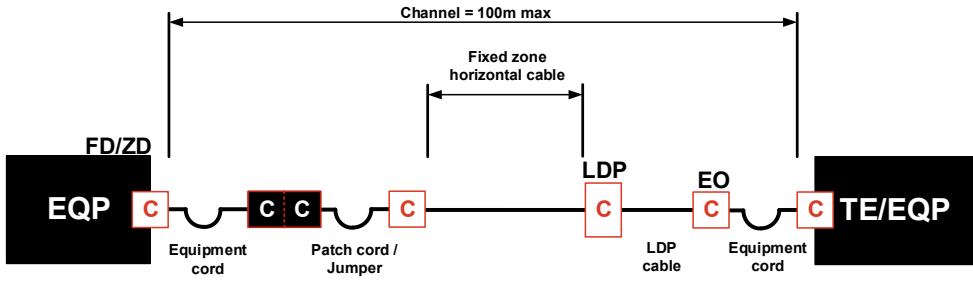
Cross connect LDP EO modèle avec un coupleur RJ45
