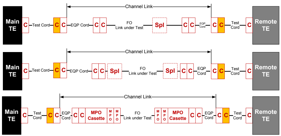
Configuration du test FO Channel
