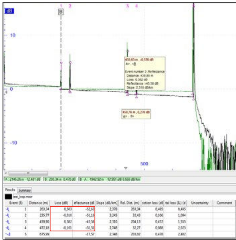
Mesure en boucle unidirectionnelle
