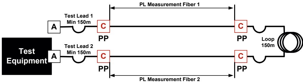
Mesure de boucle OTDR B à A
