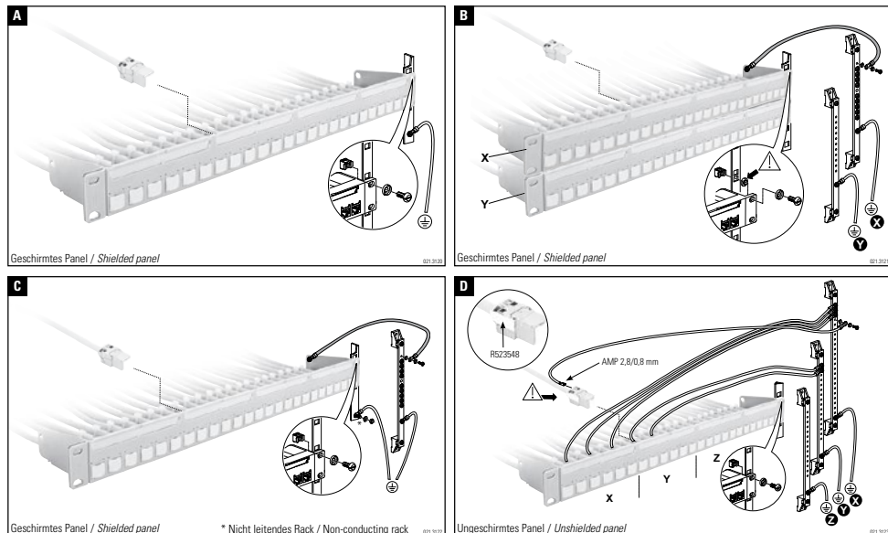
Concept de mise à la terre des panneaux R&M
