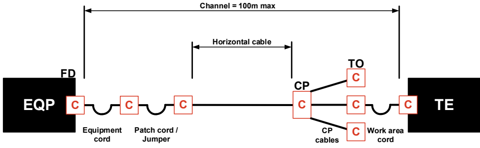
Cross connect-Modèle CP-TP
