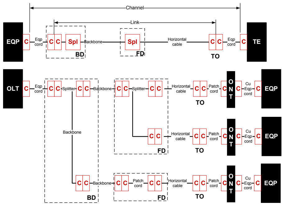
Exemple de configuration POLAN
