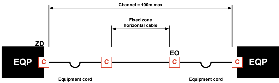
Interconnect-Modèle EO
