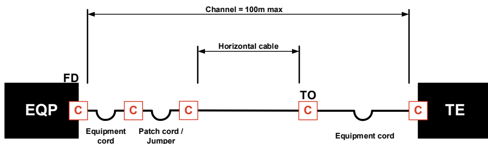
Interconnect-Modèle TO
