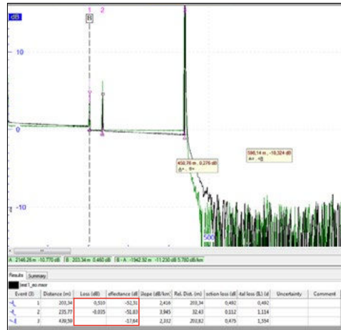
Mesure conventionnelle A vers B
