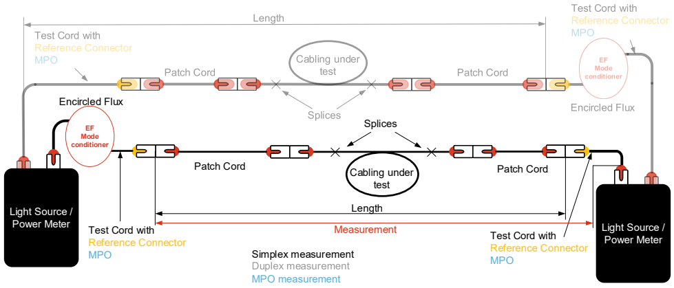
Mesure d'un CH
