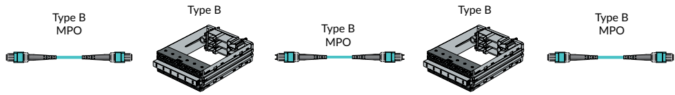
Méthode de polarité MPO R&M 40/100G Trunk B
